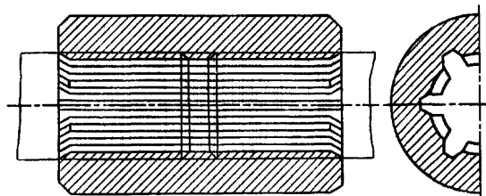
49. Втулочная муфта с прямобчными шлицами: Неразъемная муфта, которая соединяется с валами прямобчными шлицами
