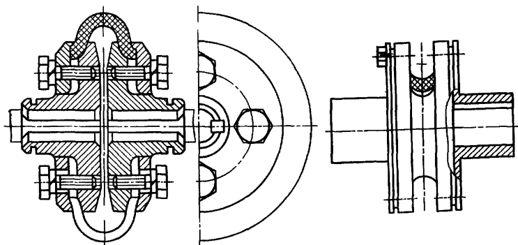
79. Упругая муфта с торообразной оболочкой: Линейная упругая муфта, которая обладает упругими и компенсирующими свойствами за счет упругой деформации неметаллической торообразной оболочки выпуклого или вогнутого профиля, установленной между торцами полумуфт
