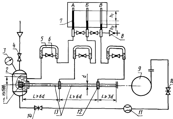
1 — испытуемое изделие; 2 — бак (4 м³); 3 — манометр; 4 — кран; 5 — демпфер; 6 — кран; 7 — пьезометры; 8 — проливочный кран; 9 — центробежный насос; 10, 14 — задвижки; 11 — расходомер; 12 — уравнивательная камера; 13 — мерный участок
