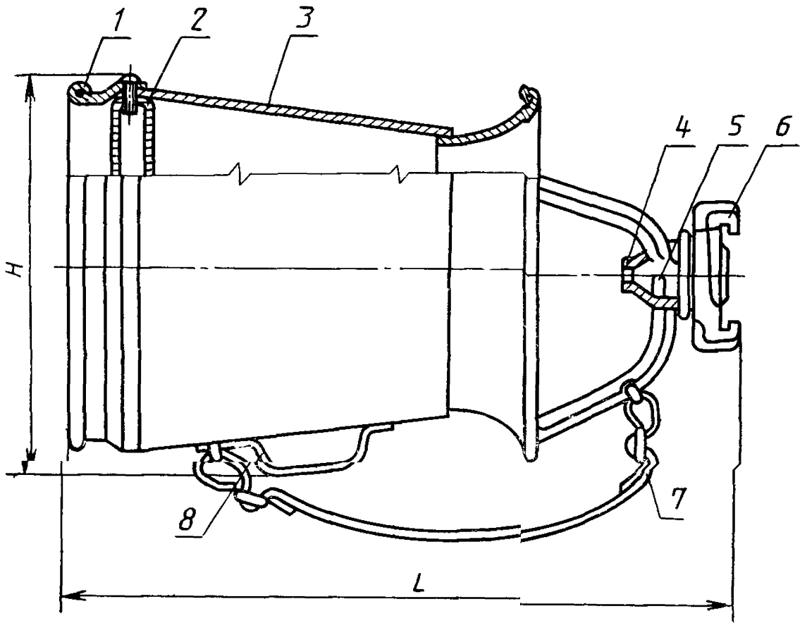
1—насадок; 2—кассета сеток; 3—корпус генератора; 4—корпус распылителя; 5—распылитель; 6—соединительная головка ГМ-70; 7—ремень; 8—ручка
