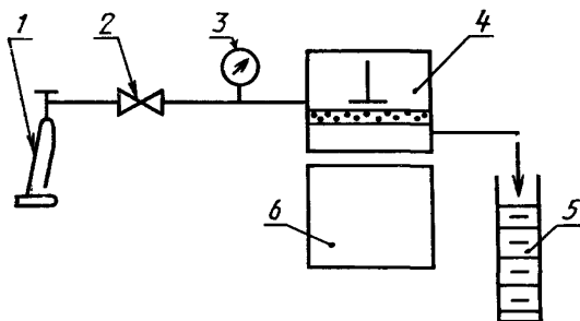
Установка для проведения испытаний
