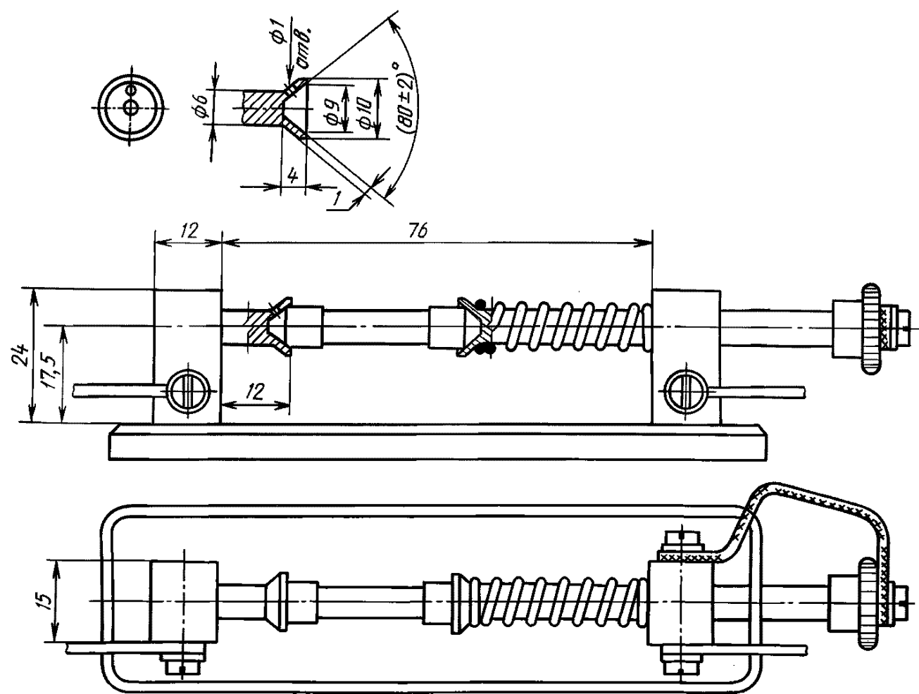
Размеры в миллиметрах. Пред. откл. 0,1 мм. Рисунок 2 — Цоколь для испытания плавких вставок размером 6,3×32 мм. Номинальные токи св. 10 А (см. 4.3.1)
