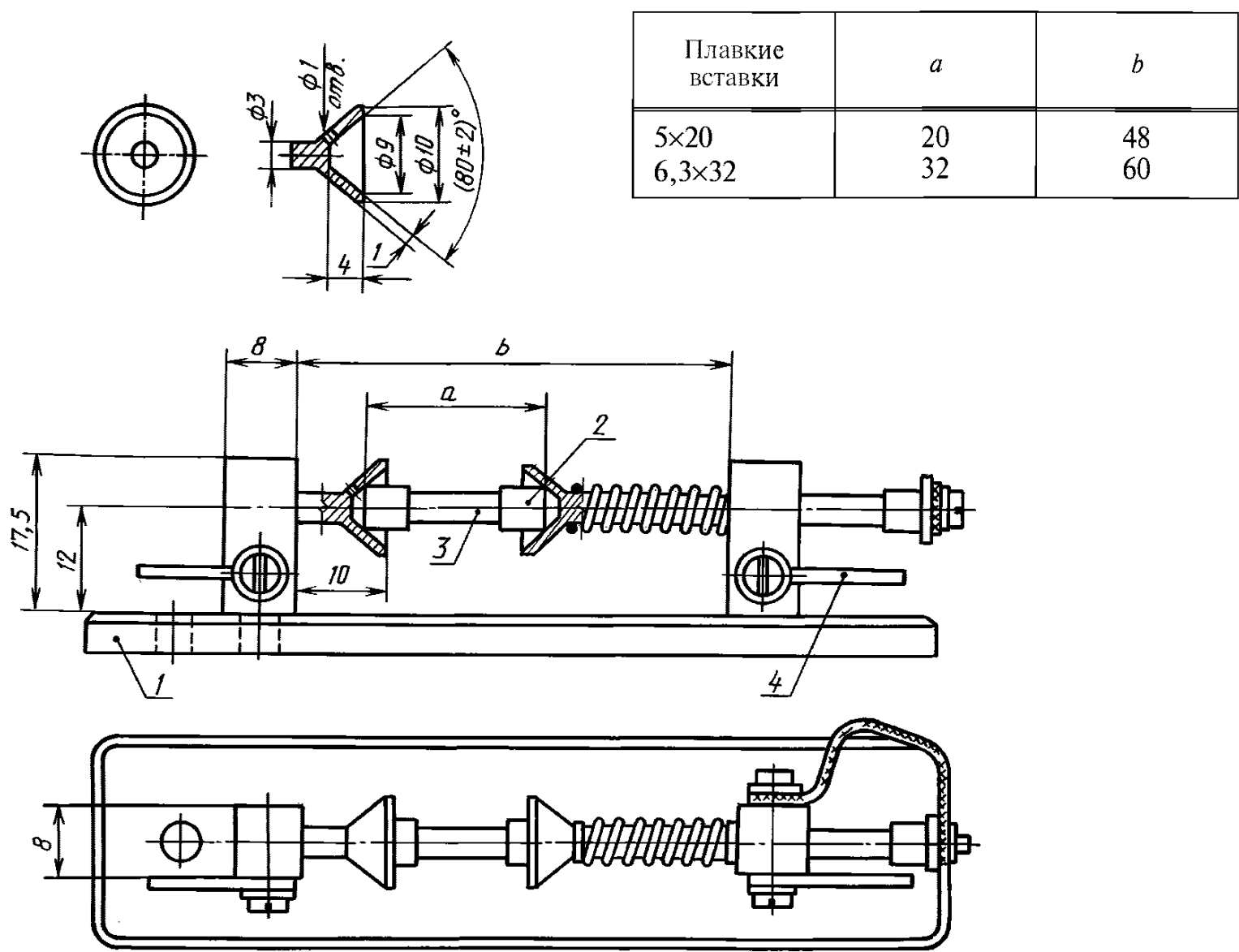
Размеры в миллиметрах. Пред. откл. 0,1 мм. 1 — цоколь из изоляционного материала с низкой теплопроводностью; 2 — контакт (наконечник) плавкой вставки; 3 — плавкая вставка; 4 — соединительный провод Рисунок 1 — Цоколь для испытания плавких вставок размером 5×20 мм и 6,3×32 мм. Номинальные токи до 10 А включ. (см. 4.3.1)
