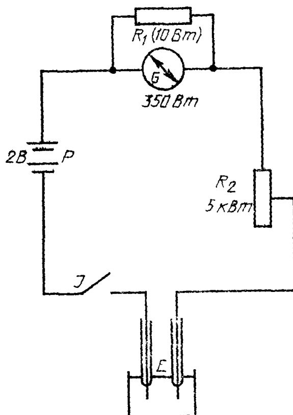
Цепь электрометрического устройства для обнаружения конечной точки P — батарея J — выключатель F — платиновые электроды, R 1 и R 2 — реостаты, G — гальванометр
