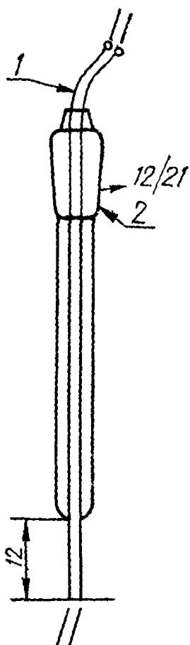
Платиновые электроды: 1 — медные проволоочки, одна из которых изолирована пластиковой оболочкой, 2 — коническое соединение из стекла, стандарт 12/21
