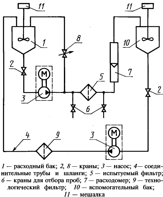
Схема стенда для определения коэффициента отсева фильтрации
