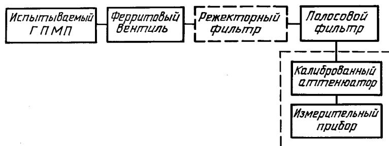
Рисунок Б.1 — Структурная схема измерений мощности побочных колебаний в испытательном тракте
