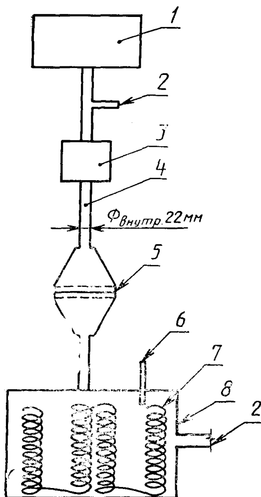
1 — аппарат ИВЛ для оживления; 2 — отвод для измерения давления; 3 — расходомер; 4 — жесткий трубопровод; 5 — имитатор сопротивления (от R 5 до R 1000); 6 — гермометр; 7 — медная проволока; 8 — имитатор растяжимости (от C 1 до C 50)
