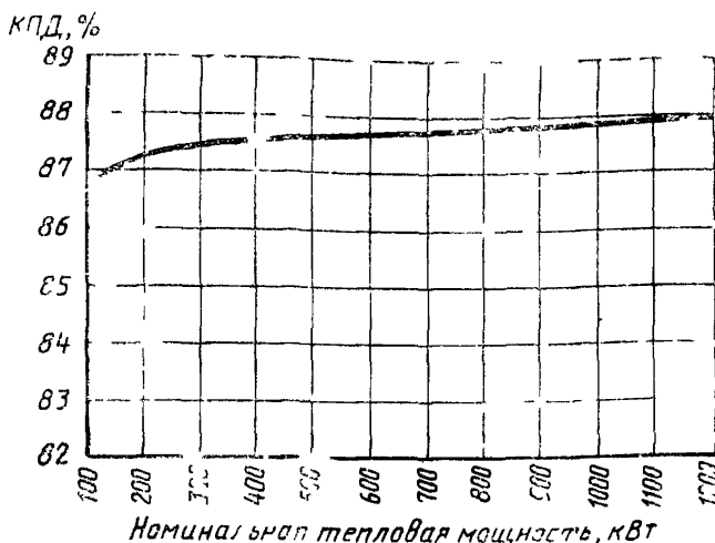
Рисунок 1 — График зависимости КПД рекуперативных воздухонагревателей от номинальной тепловой мощности
