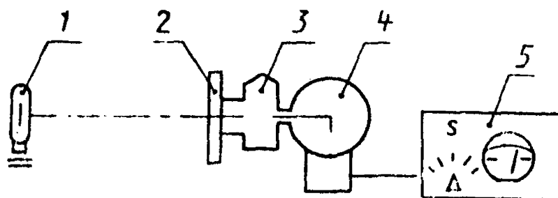
1 — нормированный источник света; 2 — молочное стекло; 3 — испытуемый фотоаппарат; 4 — светоприемный блок; 5 — контрольно-измерительный прибор
