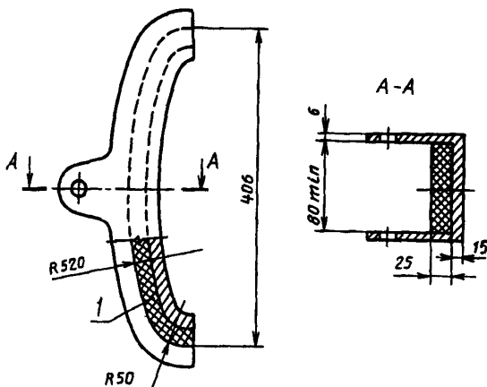
Рисунок 2 — Нагружающий блок
