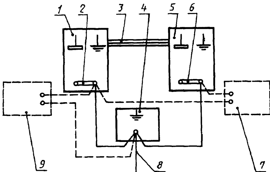
1 — первая стойка испытываемого ТС АС-ЯРО; 2, 6 — переключки между сигнальной и защитной системами заземления в стойке; 3 — линии связи между стойками; 4 — опорный узел заземления ТС АС-ЯРО; 5 — n -я стойка испытываемого ТС АС-ЯРО; 7 — подключение ИГ к зажимам защитного заземления двух стоек; 8 — цепь связи с физической землей; 9 — подключение ИГ к зажиму защитного заземления стойки и к опорному узлу заземления
