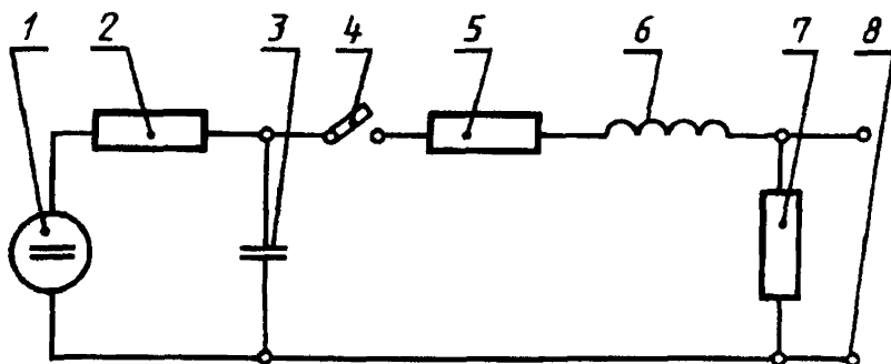
1 — источник высокого напряжения; 2 — зарядный резистор; 3 — зарядный конденсатор; 4 — коммутирующий ключ; 5 — резистор цепи формирования длительности импульса, определяющий внутреннее сопротивление ИГ; 6 — индуктивность цепи формирования длительности фронта импульса; 7 — резистор цепи формирования длительности импульса; 8 — к испытуемой цепи ТС АС-ЯРО
