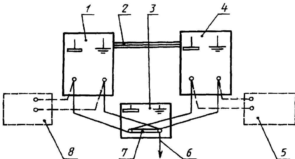
1 — первая стойка испытываемого ТС АС-ЯРО; 2 — линии связи между стойками; 3 — опорный узел заземления ТС АС-ЯРО; 4 — n -я стойка испытываемого ТС АС-ЯРО; 5 — подключение ИГ к n -й стойке испытываемого ТС АС-ЯРО; 6 — цепь связи с физической землей; 7 — перемычка между сигнальной и защитной системами заземления; 8 — подключение ИГ к первой стойке испытываемого ТС АС-ЯРО
