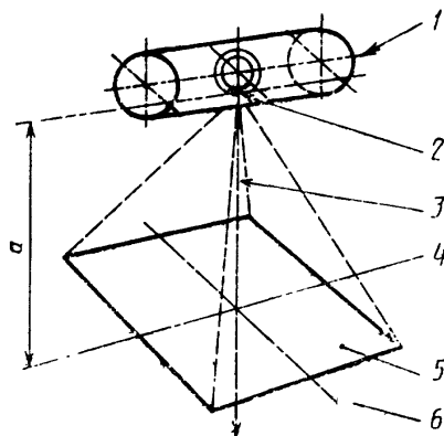
1 — продольная ось БЛОКА ИСТОЧНИКА РЕНТГЕНОВСКОГО ИЗЛУЧЕНИЯ или РЕНТГЕНОВСКОГО ИЗЛУЧАТЕЛЯ; 2 — ФОКУСНОЕ ПЯТНО; 3 — ОПОРНАЯ ОСЬ; 4 — основная ось X ; 5 — нормированное максимальное симметричное РАДИАЦИОННОЕ ПОЛЕ; 6 — основная ось Y ; a — РАДИАЦИОННОЕ ПОЛЕ
