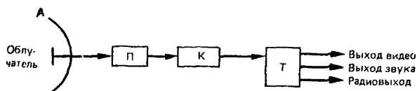
Рисунок 1 — Структурная схема установки индивидуального приема
