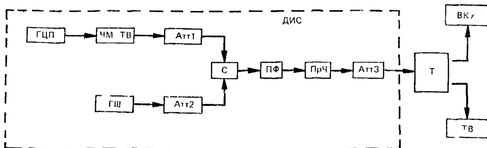
Рисунок 10 — Структурная схема измерения «динамического порога»
