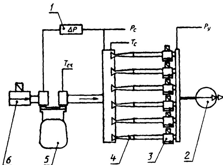
1 — дифманометр измерения потери давления \Delta P на счетчике; 2 — вакуумный насос; 3 — выходные краны сопел; 4 — образцовое звуковое сопло; 5 — испытуемый счетчик; 6 — входной кран установки; T_{сч} — температура на выходе испытуемого счетчика; T_c — температура на входе сопла; P_c — давление на входе сопла; P_y — давление на выходе сопла
