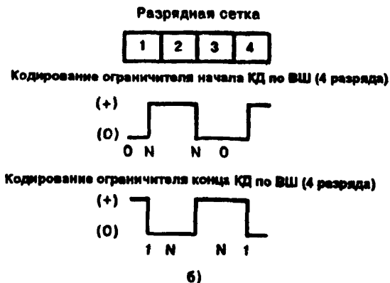
Рисунок 8 — Кодирование синхροпреамбулы и ограничителей начала и конца КД
