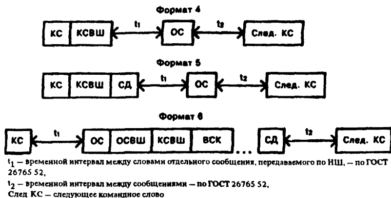
Рисунок 10 — Форматы сообщений для передачи команд управления обменом и контроля состояния по ВШ в режиме «команда-ответ»
