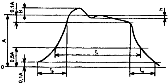
Рисунок 12 — Форма сигнала оптического излучения в ВОСРП
