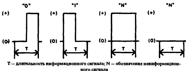
Рисунок 3 — Представление информации в ВШ
