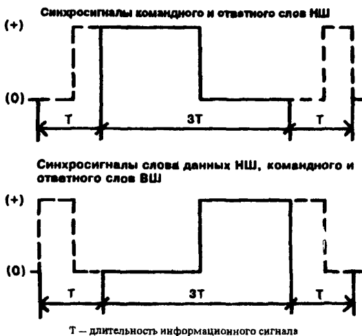
Рисунок 4 — Представление синхросигналов слов, передаваемых по НШ, при использовании ВОСПР
