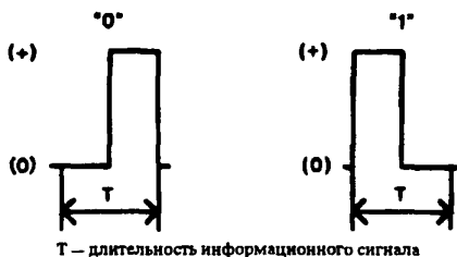
Рисунок 2 — Представление информации в НШ при использовании ВОСРП
