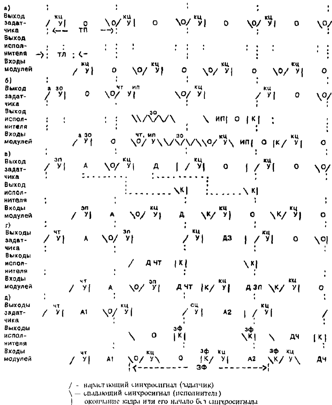
Рисунок Б.8 — Синхронизация и кодирование битов информации на последовательной магистрали
