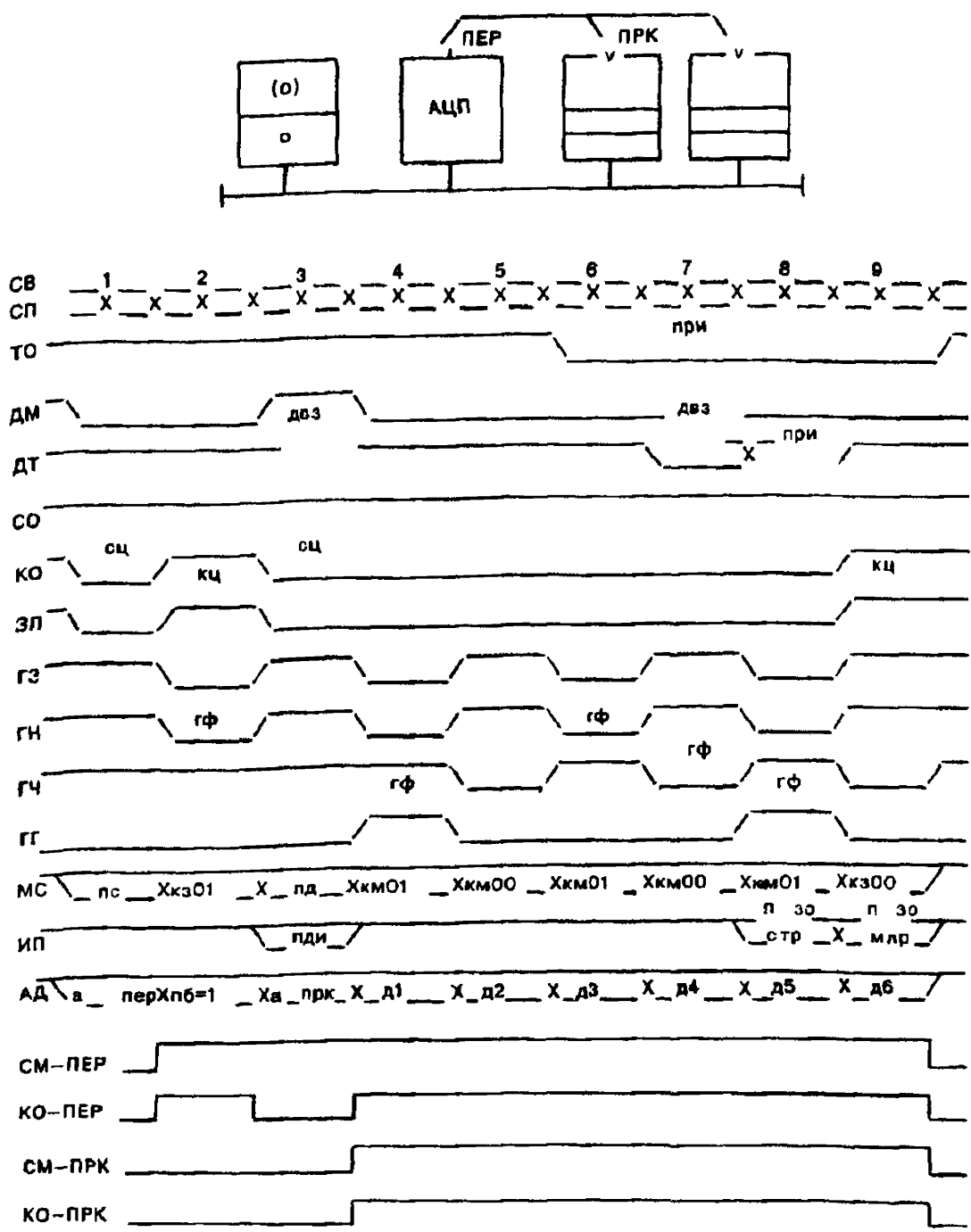
Рисунок Б.7 — Временные диаграммы сигналов в двухадресном групповом цикле передачи с расслоением памяти, в течение которого также проходит арбитраж ЗО
