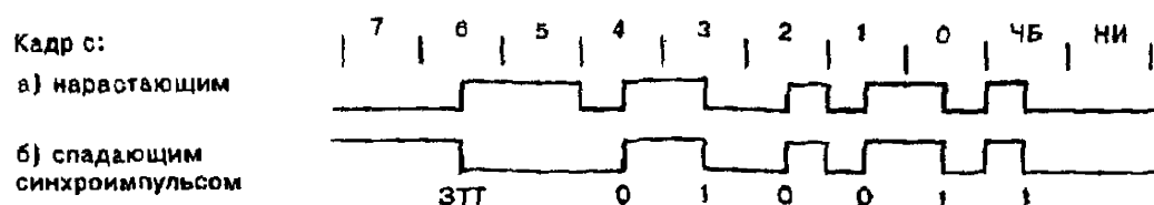
Рисунок Б.8 — Синхронизация и кодирование битов информации на последовательной магистрали
