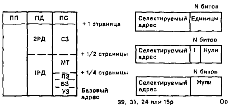
Рисунок Б.10 — Расположение регистров в зоне ВА модуля
