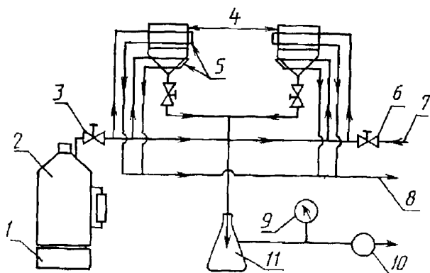
1 -- источник н-пирева 2 - генератор пара 3 - пар 4 - фильтровальный блок 5 - охлаждающие трубки 6 - холодная вода 7 - подвод охлаждающей смеси 8 - фенольная тиния 9 - вакуумный манометр 10 - вакуумный насос 11 - колба Бюхнера
