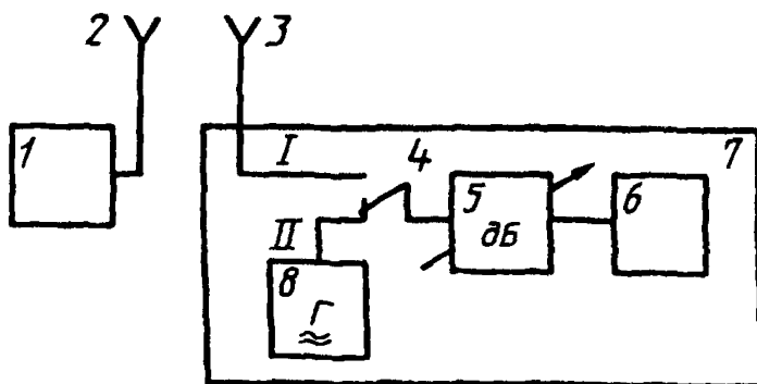
1 — контролируемый радиопередатчик; 2 — антенно-фидерная система; 3 — измерительная антенна; 4 — коаксиальный переключатель; 5 — аттенюатор; 6 — измерительный приемник; 7 — экранированная камера (используется при необходимости); 8 — измерительный генератор
