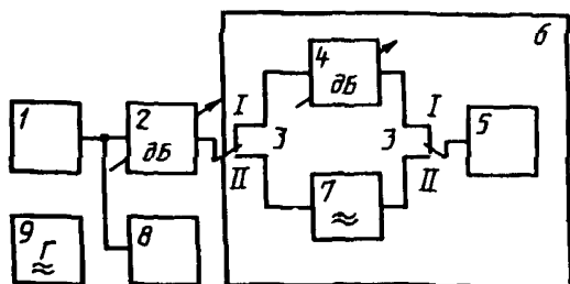
1 — контролируемый радиопередатчик, 2 — развязывающий аттенюатор, 3 — высокочастотный переключатель, 4 — измерительный аттенюатор, 5 — измерительный приемник, 6 — экранированная камера (используется при необходимости), 7 — фильтр, 8 — эквивалентное нагрузочное сопротивление, 9 — генератор сигналов низкочастотный
