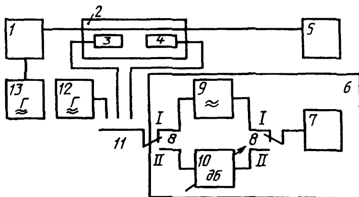
1 — контролируемый передатчик, 2 — направленный ответвитель, 3, 4 — измеритель мощности соответственно падающей и отраженной волн, 5 — антенна, 6 — экранированная камера (используется при необходимости), 7 — измерительный приемник, 8, 11 — высокочастотные переключатели, 9 — измерительный аттенюатор, 10 — фильтр (используется при необходимости), 12 — измерительный генератор, 13 — генератор сигналов низкочастотный
