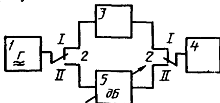
1 — измерительный генератор; 2 — высокочастотный переключатель; 3 — измерительный тракт (начиная с выхода направленного ответвителя или делителя, или измерительной антенны); 4 — измерительный приемник; 5 — измерительный аттенюатор
