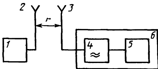
1 — контролируемый радиопередатчик; 2 — антенно-фидерная система; 3 — измерительная антенна; 4 — фильтр; 5 — измеритель напряженности поля; 6 — экранированная камера (используется при необходимости)
