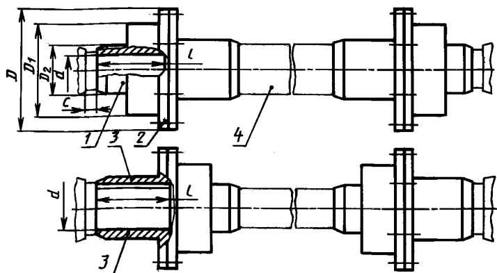
Исполнение 1 Варианты сборки
