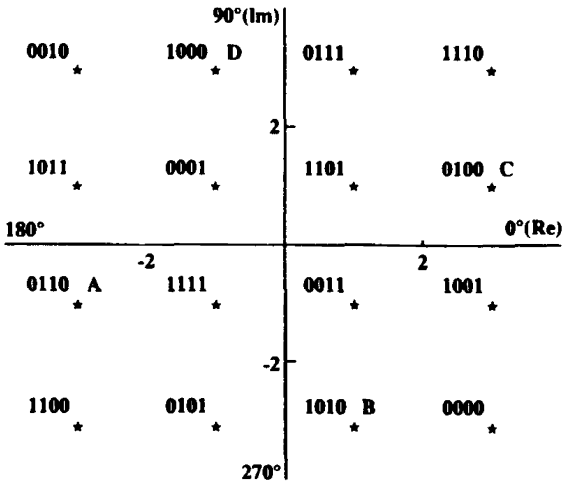
Рисунок 2 — Сигнальное созвездие КАМ-32 для скорости 9600 бит/с
