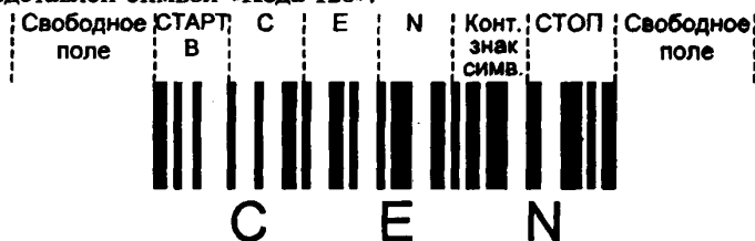
Рисунок 1 — Символ «Кода 128», кодирующий знаки CEN
