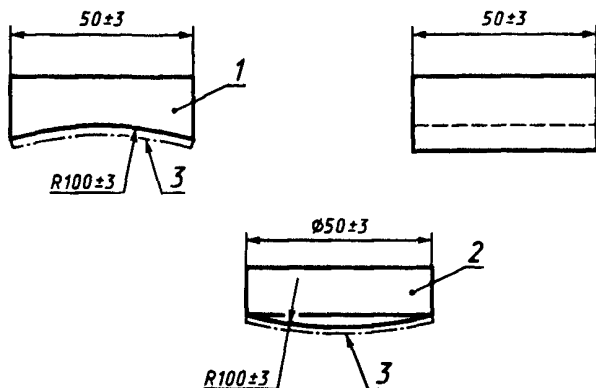
Рисунок 1 — Нагружающие пластины
