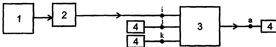
Рисунок В.5 — Схема измерения КСВН с помощью панорамного измерителя
