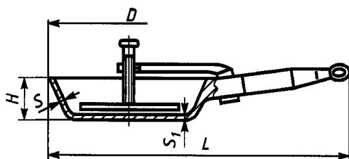
Рисунок 8 — Сковорода для приготовления цыплят-табака
