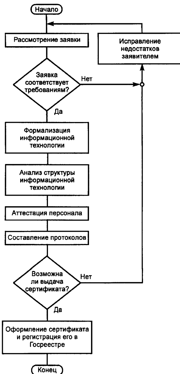
Рисунок А.2 — Блок-схема алгоритма процедуры аттестации информационной технологии в области качества служебной информации
