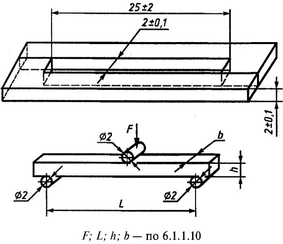
Рисунок 1 — Форма и приспособление для испытания на изгиб
