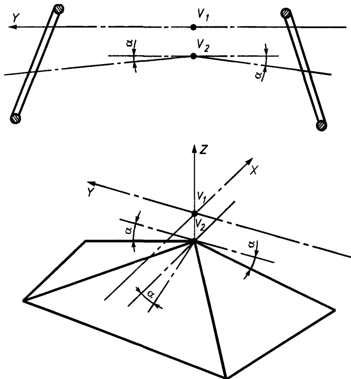
Рисунок 8 — Расположение плоскостей, являющихся границами нормативного поля обзора \Pi
