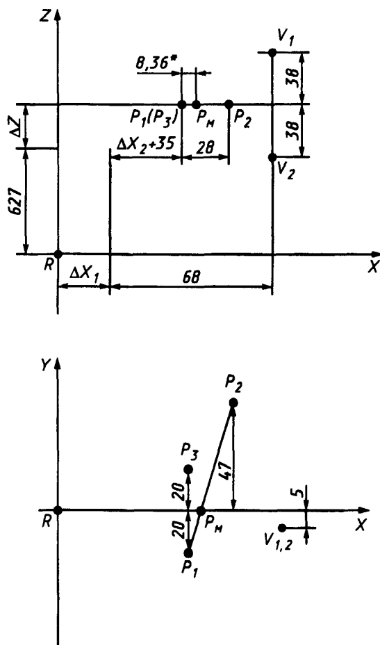
Рисунок 3 — Определение координат точек V и P
