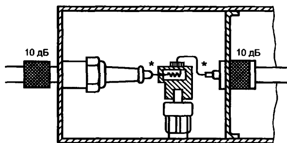
Рисунок В 10 — Помехоподавляющий ротор распределителя
