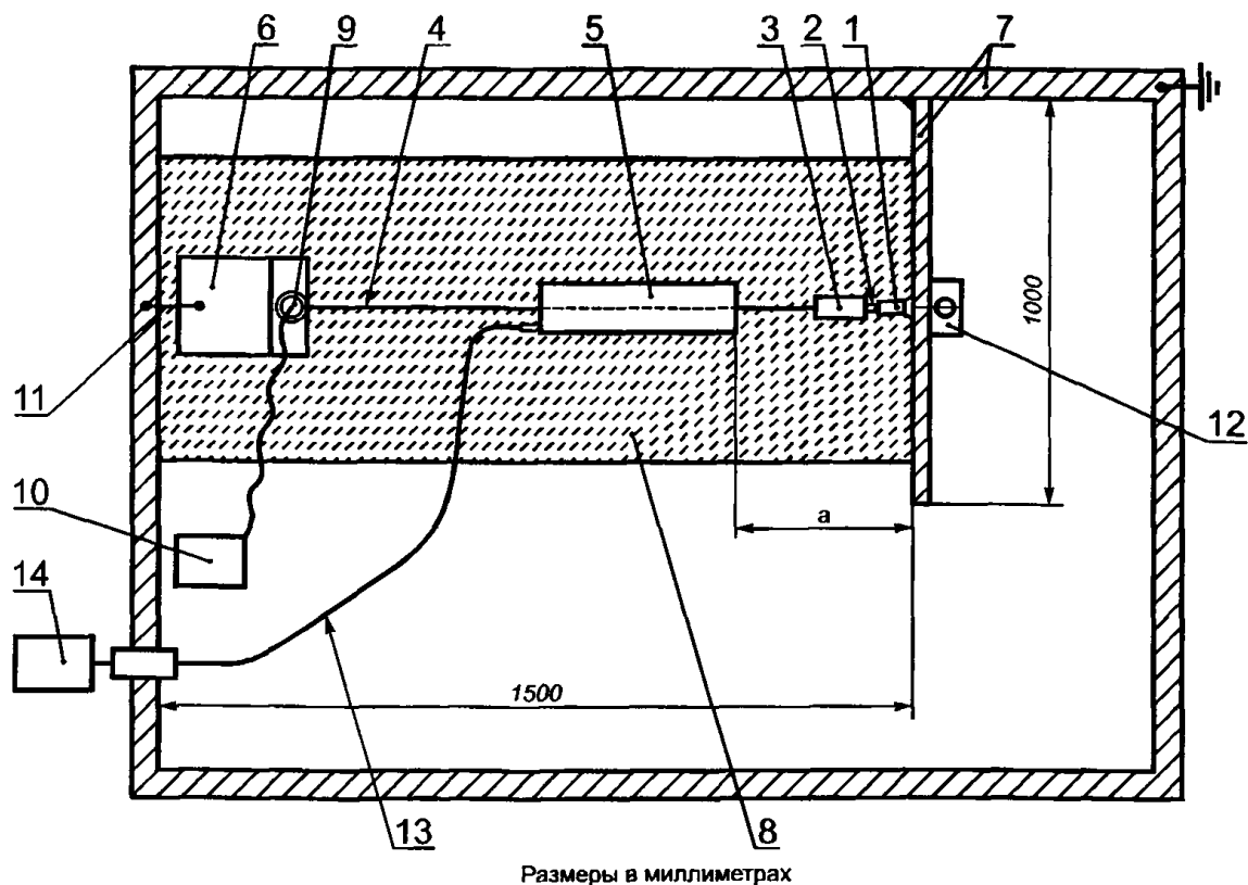
Рисунок Г 2 — Испытательная установка, вид сверху
