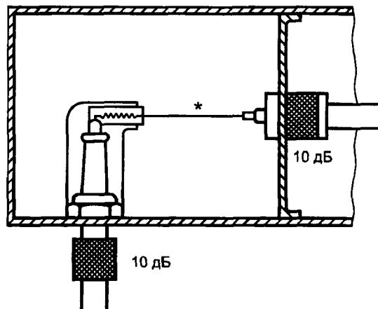
Рисунок В 6 — Правоугольное помехоподавляющее устройство системы зажигания со свечей зажигания (экранированное или неэкранированное)
