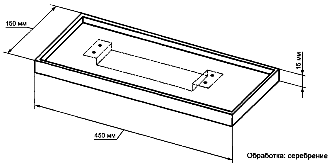
Рисунок В.3 — Детали крышки испытательного контейнера
