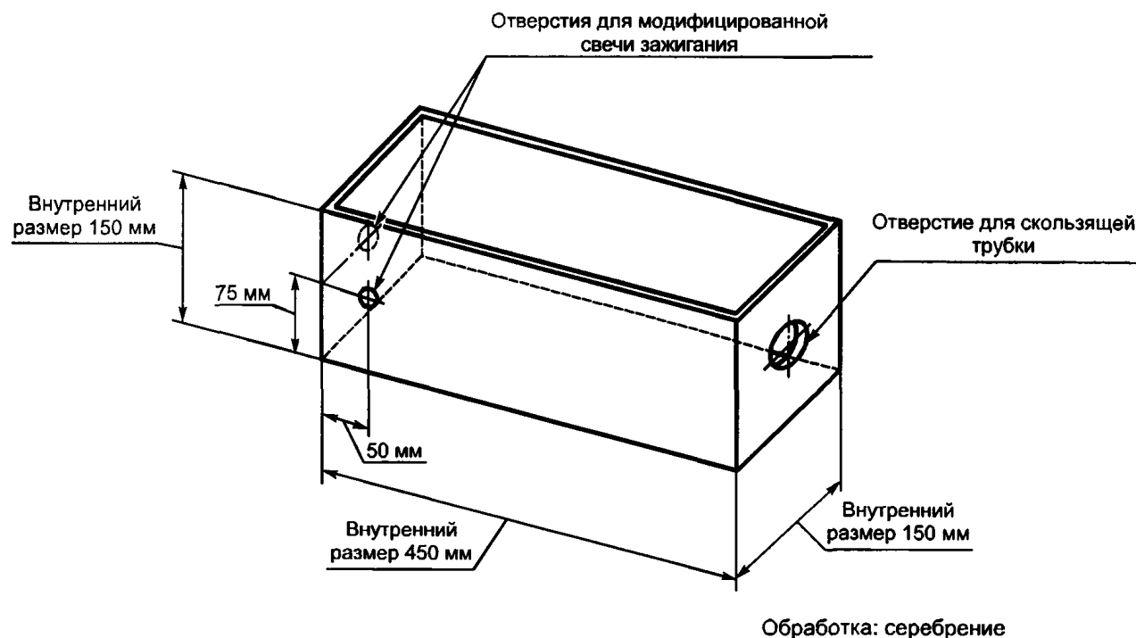
Рисунок В.4 — Размеры испытательного контейнера
