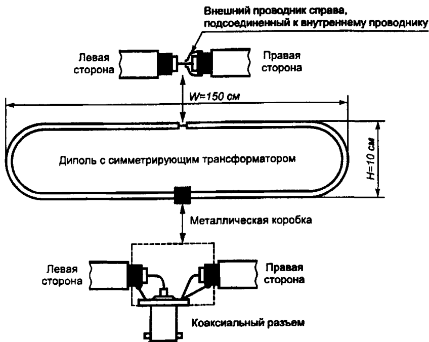
Рисунок Д.3 — Конструкция калибровочного диполя
