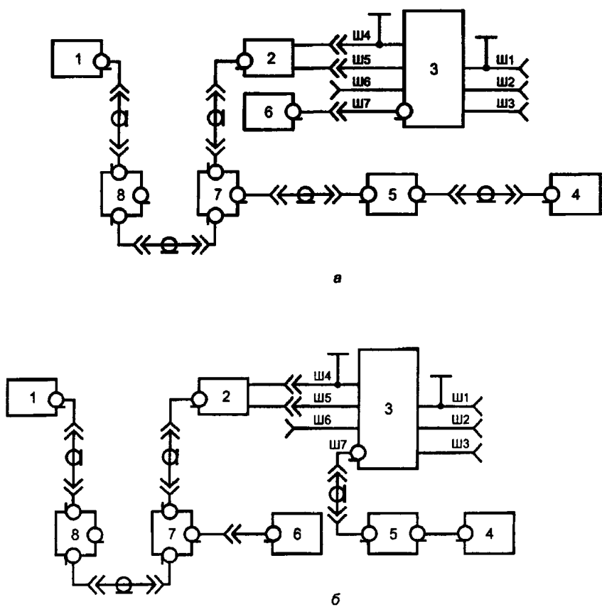
а — схема измерения напряжения на входе V-образного эквивалента сети; б — схема измерения напряжения на выходе V-образного эквивалента сети
