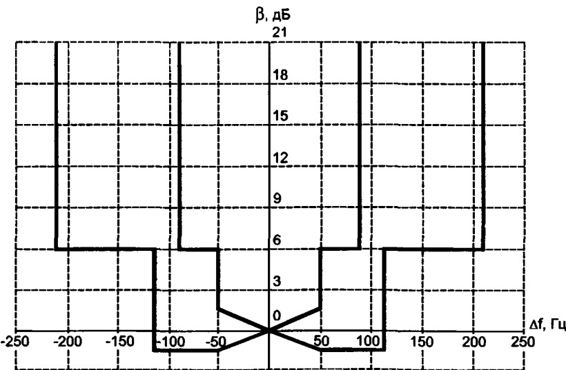
Рисунок 1 — Пределы характеристики избирательности измерителя ИРП в полосе частот от 0,009 до 0,15 МГц
