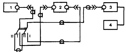
1 — генератор синусоидальных сигналов; 2 — режекторный фильтр; 3 — аттенюатор; 4 — вольтметр переменного тока
