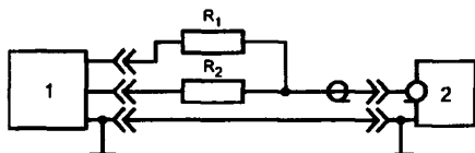
Рисунок 10 — Схема проверки степени симметрии симметричного входа измерителя ИРП
