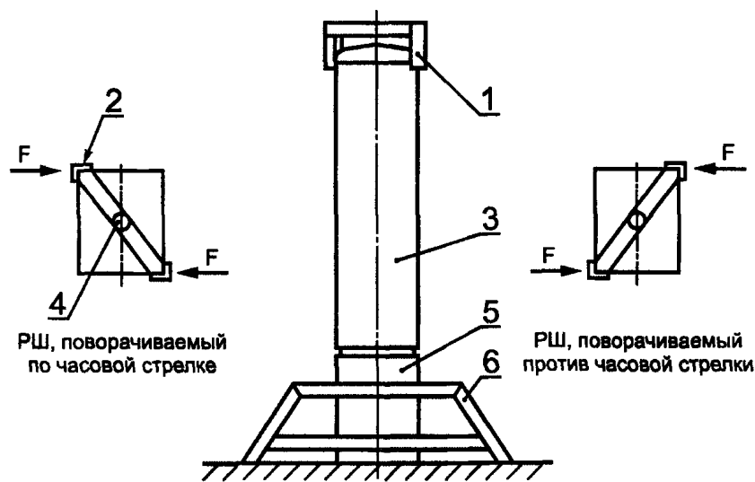
1 — вращающееся устройство, устанавливаемое на РШ; 2 — уголок 60 × 60 × 5 мм длиной 100 мм; 3 — РШ; 4 — центр вращения; 5 — основание; 6 — опора; F = 1000\text{ Н}
