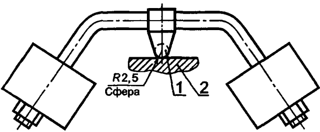
1 — стальной шарик; 2 — образец Рисунок 14 — Установка для испытания прочности материалов при нагревании
