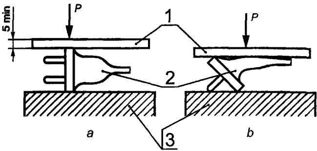
P — усилие 150 Н; 1 — стальная нажимная пластина; 2 — образец; 3 — стальное основание Рисунок 12 — Установка для испытания на сжатие
