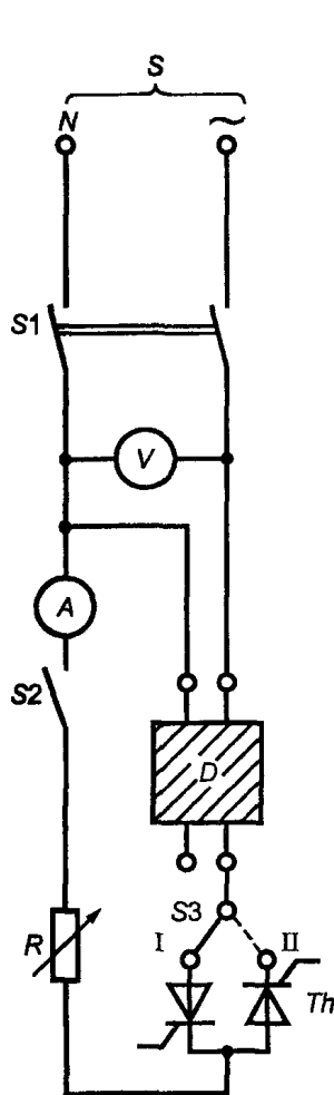
S — источник электрической энергии; V — вольтметр; A — амперметр, показывающий среднее квадратическое значение; D — испытуемое УЗО-ДП; R — регулируемый резистор; Th — тиристор; S1 — двухполюсный выключатель; S2 — однополюсный выключатель; S3 — однополюсный выключатель на два направления
