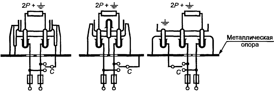
Рисунок 8 — Схемы соединения для испытания на нормальную работу
