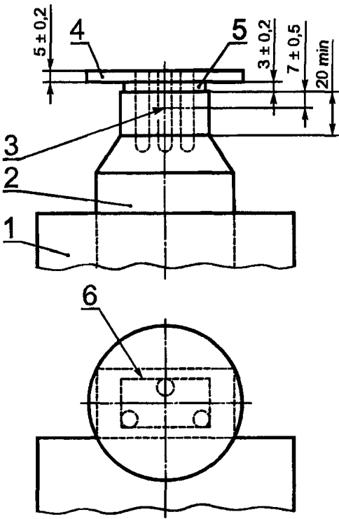
1 — нагревательный элемент; 2 — металлическая часть; 3 — термопара; 4 — изоляционная плита; 5 — прокладка; 6 — контур вилки
