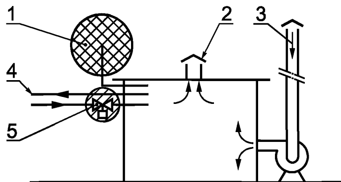
1 — вытяжная труба отбора проб; 2 — выход воздуха из помещения; 3 — вход воздуха для вентиляции; 4 — контуры отбора проб; 5 — запорный кран
