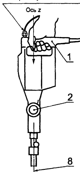
Рисунок 1 — Направление измерений; положение и крепление датчика
