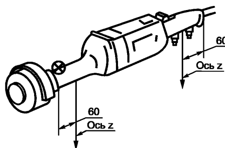
в) Прямая шлифовальная машина
