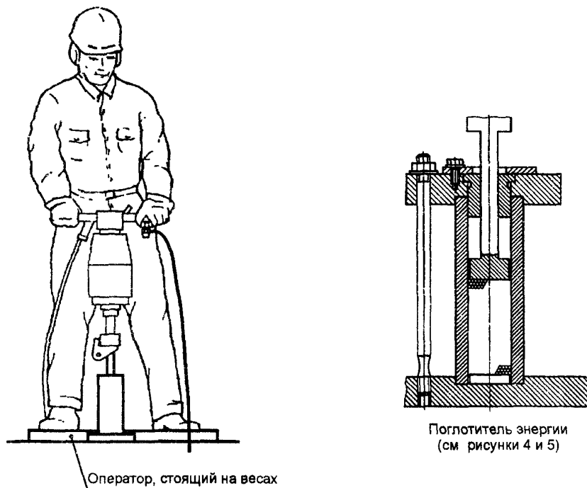
Рисунок 2 — Рабочее положение оператора при испытаниях бетонолома
