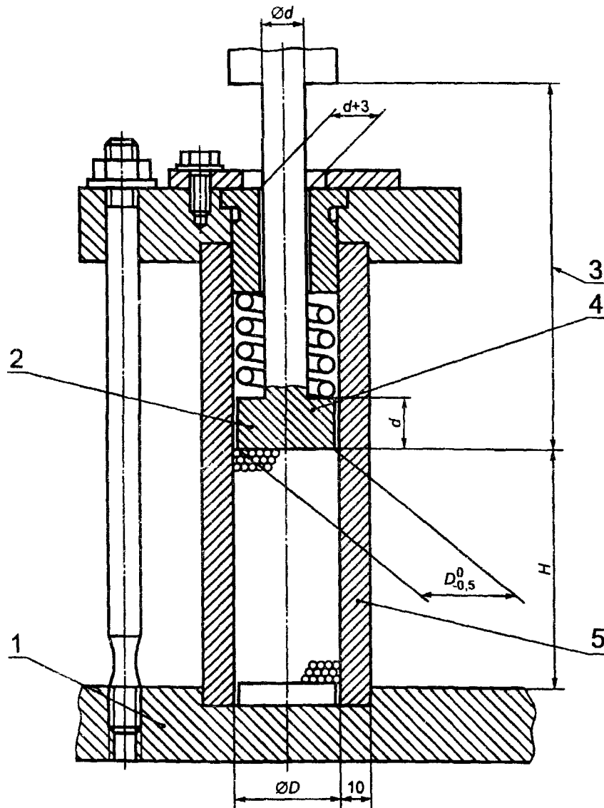
1 — бетонный блок массой не менее 300 кг; 2 — оптимальная конструкция наконечника испытательного инструмента, действующего на шарики; 3 — расстояние от торца испытуемой машины до поглощающего столба шариков; 4 — закаленная сталь твердостью (55 \pm 2) HRC; 5 — закаленная сталь твердостью (62 \pm 2) HRC
