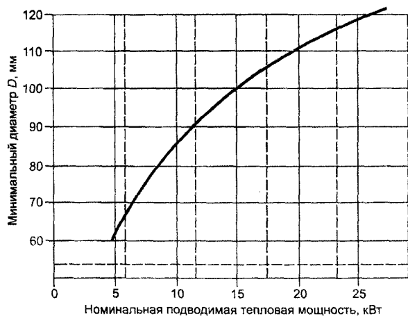
Рисунок 1 — Зависимость минимального раструса дымохода от номинальной подводимой тепловой мощности
