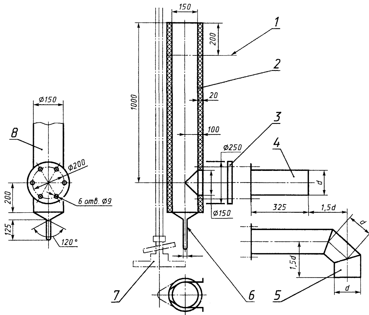
1 — плоскость измерения (пробоотборник и термопара); 2 — теплоизоляция (стекловолокно плотностью 64 кг/м 3 ); 3 — прокладка; 4, 5 — соединительные трубы из нержавеющей стали; 6 — трубка внутренним диаметром 8 мм и толщиной стенки 1 мм; 7 — опорная стойка (высота регулируемая); 8 — труба дымохода из нержавеющей стали
