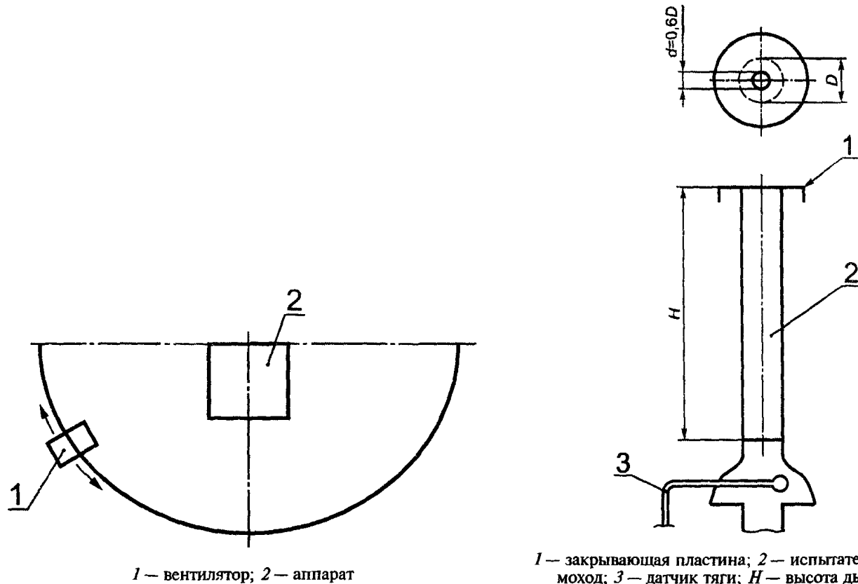
Рисунок 7 — Расположение оборудования для испытаний на ветроустойчивость
