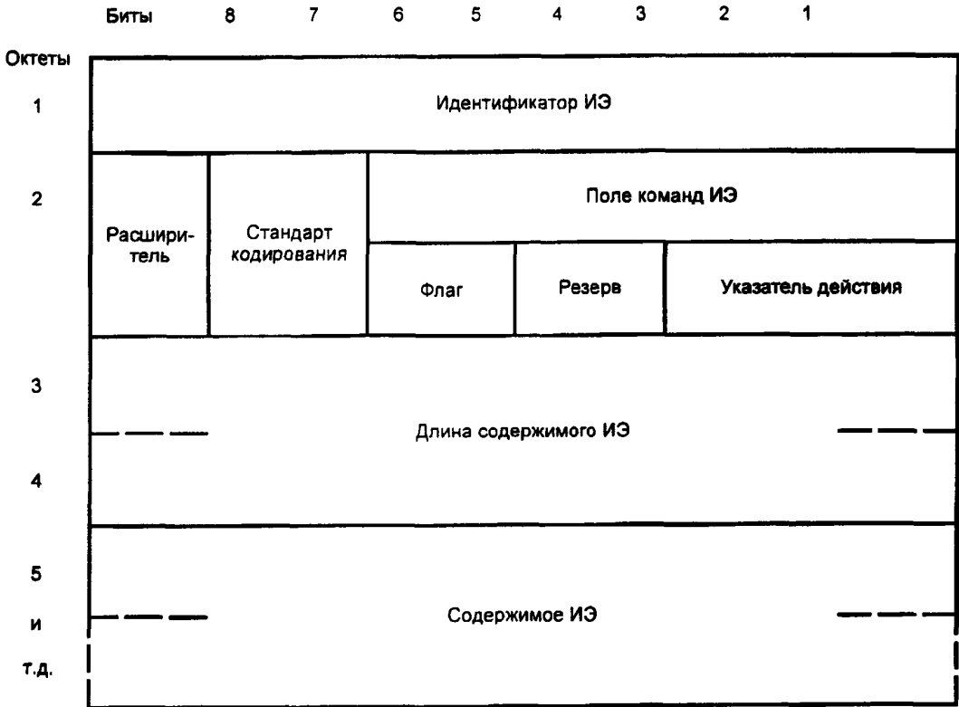
Рисунок 3 — Структура формата ИЭ
