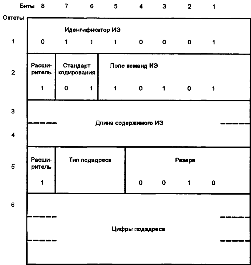
Рисунок 10 — Формат ИЭ «Субадрес вызываемой стороны»
