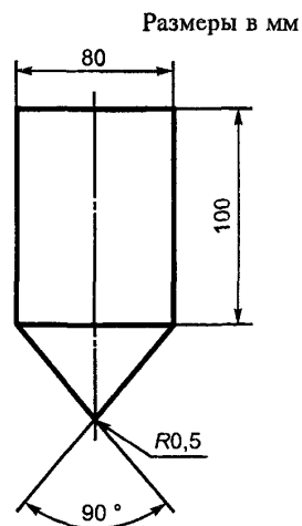
Рисунок 6 — Испытательный конус
