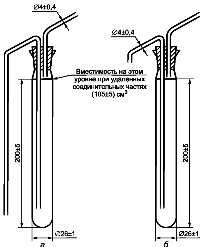
a — с соединительными частями сифона; б — с соединительными частями промывного типа
