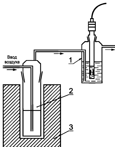
1 — измерительная ячейка; 2 — аэрационный сосуд; 3 — нагревательный блок
