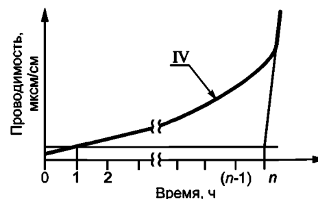
Рисунок А.1 — Примеры кривых проводимости
