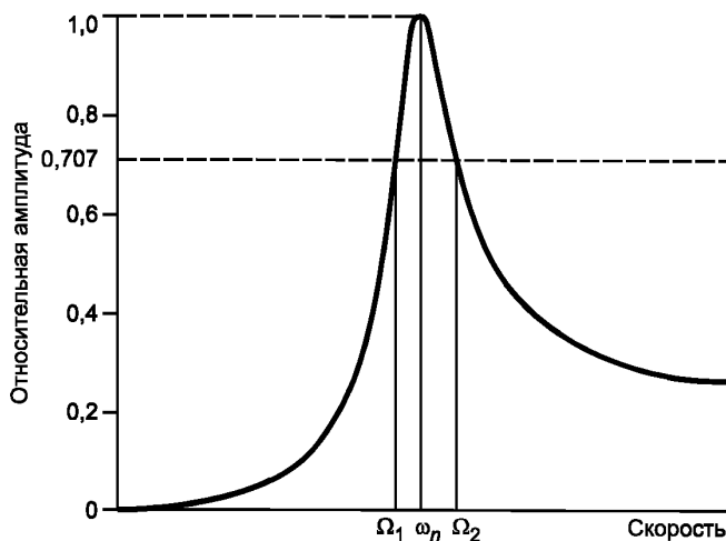
Рисунок 5 — Диаграмма Бодe для оценки модальной чувствительности
