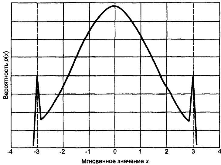
Рисунок А.3 — Негативная плотность вероятности распределения
