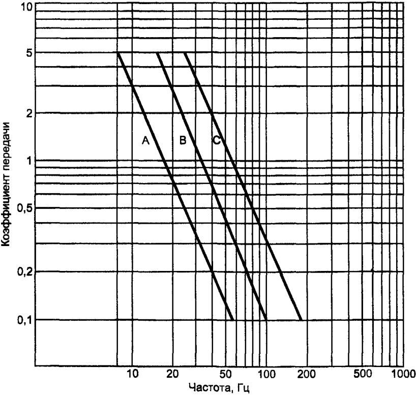
Рисунок A.6 — Коэффициент передачи виброизолятора
