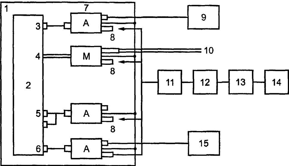
1 — пластина заземления; 2 — испытуемое оборудование; 3 — выходные зажимы; 4 — провод электропитания; 5 — зажимы для подключения кабеля блока дистанционного управления; 6 — входные зажимы; 7 — устройства связи; 8 — резистор сопротивлением 50 Ом; 9 — измеритель ИРП; 10 — к сети электропитания; 11 — аттенюатор; 12 — фильтр нижних частот; 13 — усилитель мощности (при необходимости); 14 — ГС-2; 15 — ГС-1
