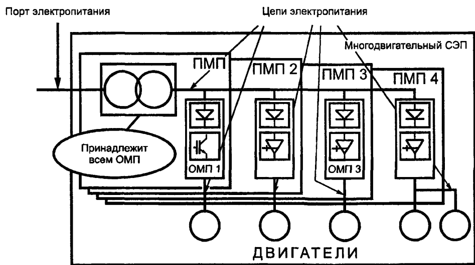
Рисунок 4 — Цели электропитания СЭП с общим входным трансформатором
