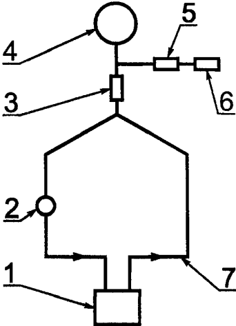
1 — аппарат ИВЛ; 2 — проверяемое устройство для измерения объема; 3 — сопротивление; 4 — модель легких; 5 — датчик давления; 6 — регистратор давления с предельной погрешностью ±2 % действительного значения для проверки точности устройства измерения объема; 7 — дыхательный контур
