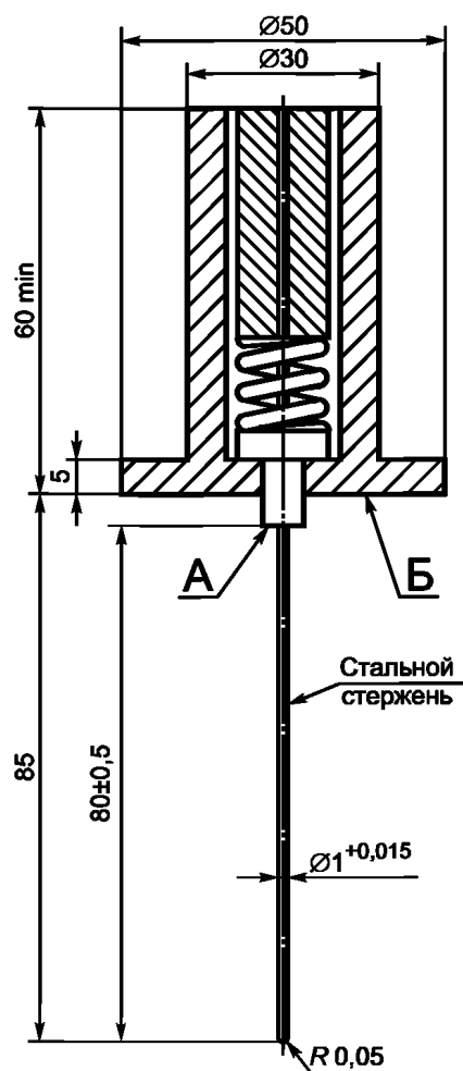
Рисунок 2 — Прибор для проверки недоступности токоведущих частей в удлинительях
