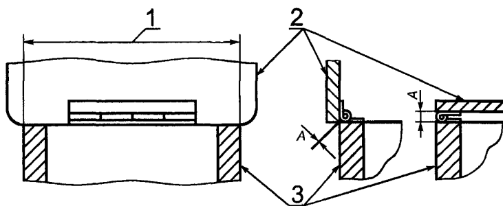
1 — шарнирная линия; 2 — крышка; 3 — ящик; A — расстояние между краями деталей, соединенных шарниром
