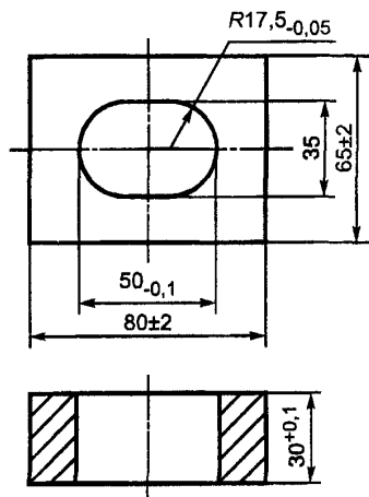
Рисунок 17 — Испытательный шаблон А
