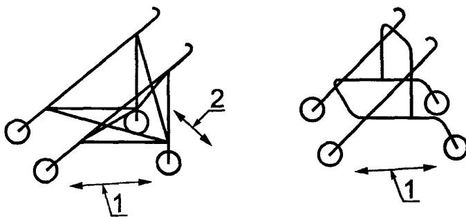
1 — движение корпуса; 2 — движение ручки
