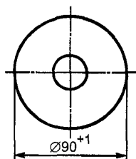
Рисунок 20 — Испытательный зонд C
