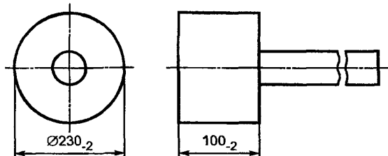
Рисунок 21 — Испытательный зонд D
